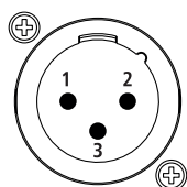
XLR插座 (公端)
