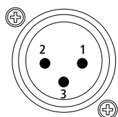
XLR插座 (母端)
